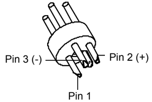
Tipo XLR balanceado
