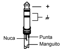
Tipo TRS no balanceado
