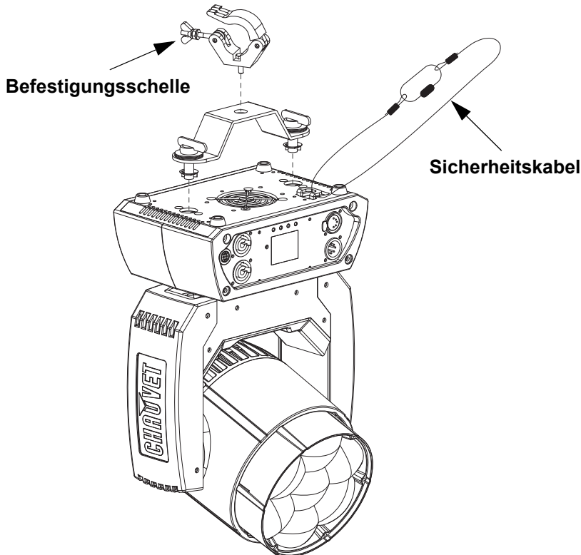
Montage über Kopf
